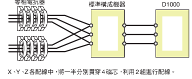
連接圖c
