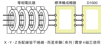
連接圖b
