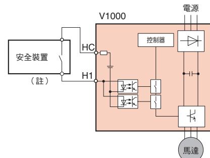
安全裝置的使用範例
