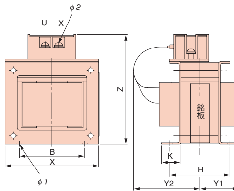
外觀圖 2
