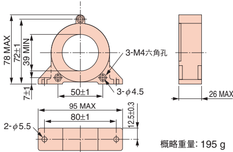
型號 F6045GB
