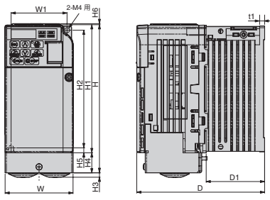
外觀圖 1
