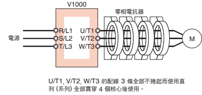
連接圖 b
