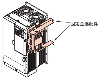
單元 (PS-V10M) 與固定金屬配件安裝完成時
