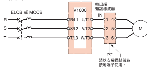
連接圖
