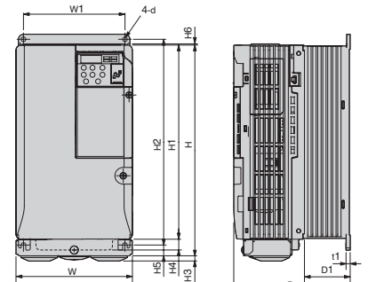
外觀圖 3
