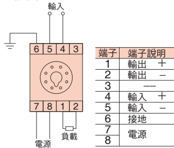
連接圖
