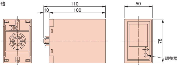
外觀尺寸 mm GP 系列本體
