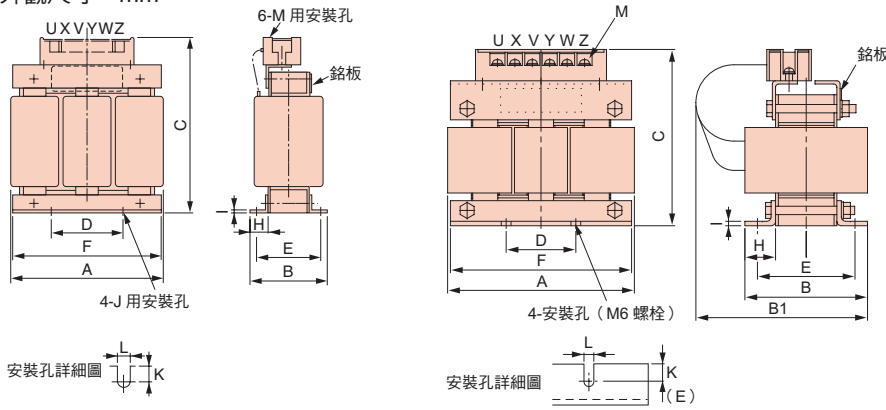
外觀圖 1
