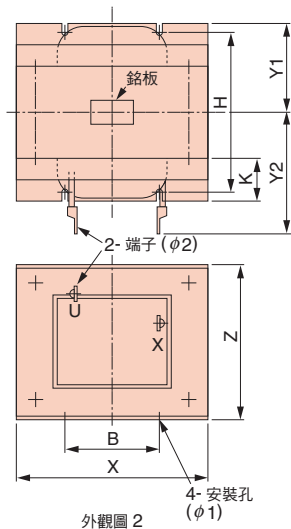
外觀圖 2
