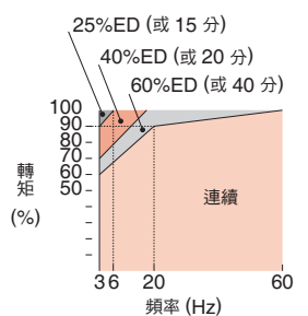
本公司標準馬達之容許負載特性
