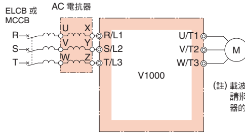
連接圖
