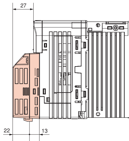
CIMR-VA2A0004 範例
