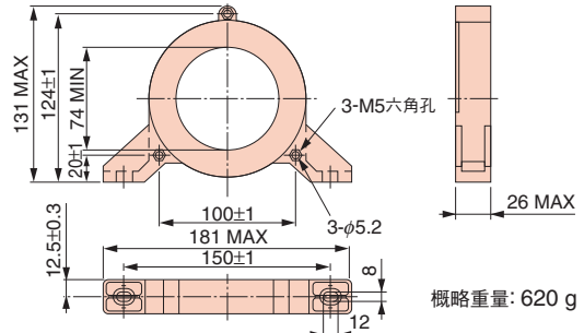
型號 F11080GB
