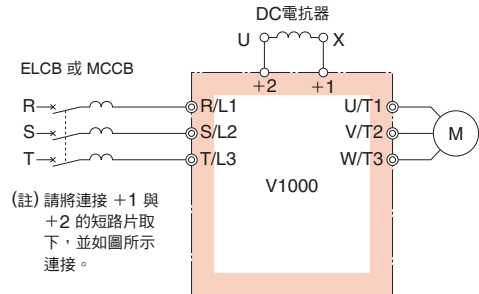
連接圖
