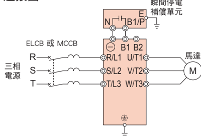
連接圖
