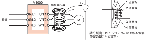
連接圖 a
