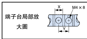
上圖為三相輸入範例。
