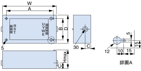
上圖為三相輸入範例。
