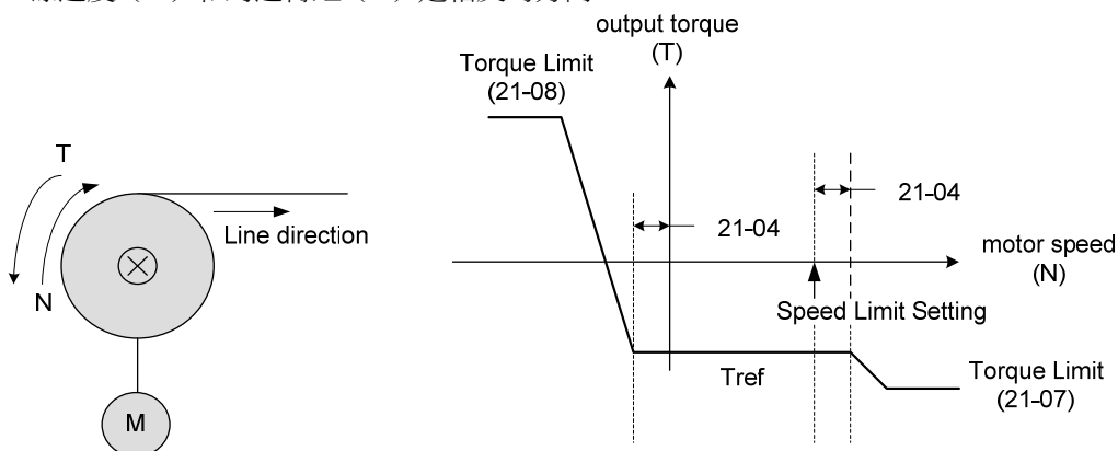
圖 4.3.125 捲出操作
