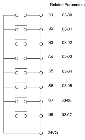
圖 4.3.16 多機能數位輸入與相關參數
