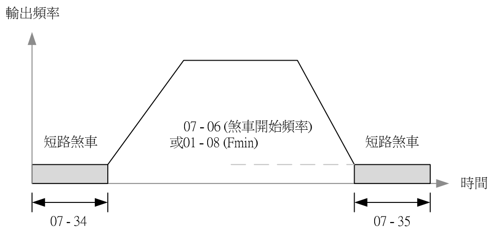
圖4.3.57b PMSLV的煞車動作
