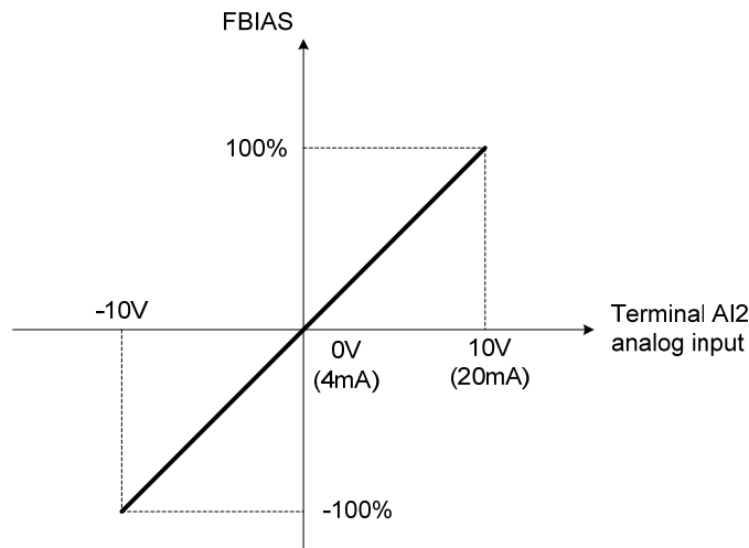
圖4.3.40 偏壓調整
