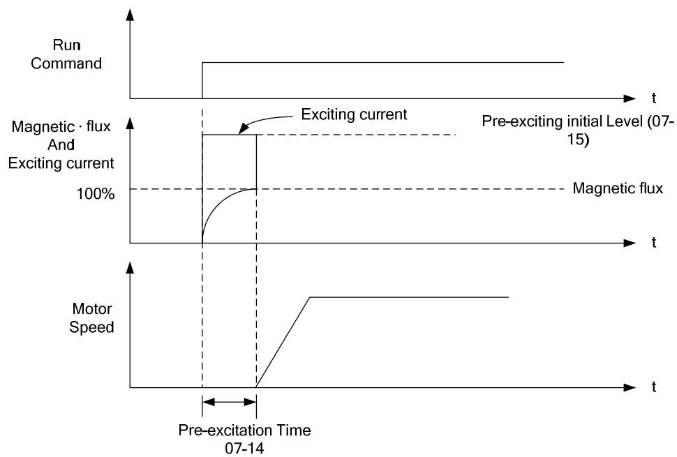
圖4.3.62 預激磁操作
