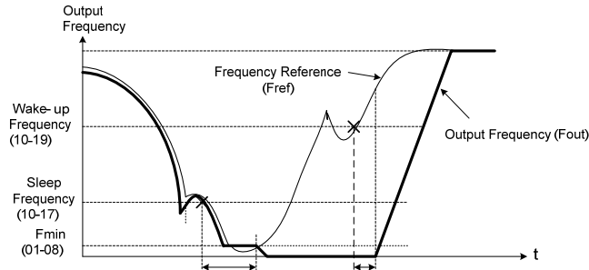
(b) PID 休眠/喚醒之時序圖
