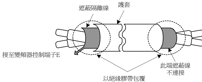
圖 3.4 隔離絞線處理情形
