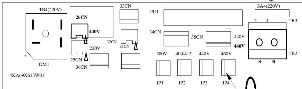
圖 3.5.1 電源電壓選擇基板
