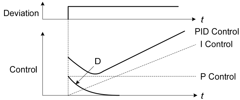
圖 4.3.77 PID 控制操作
