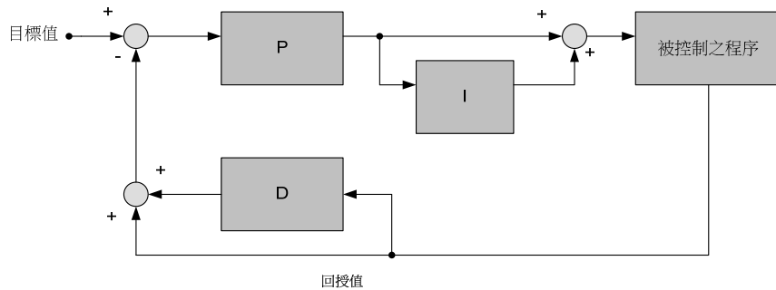
圖 4.3.78 回授微分 PID 控制
