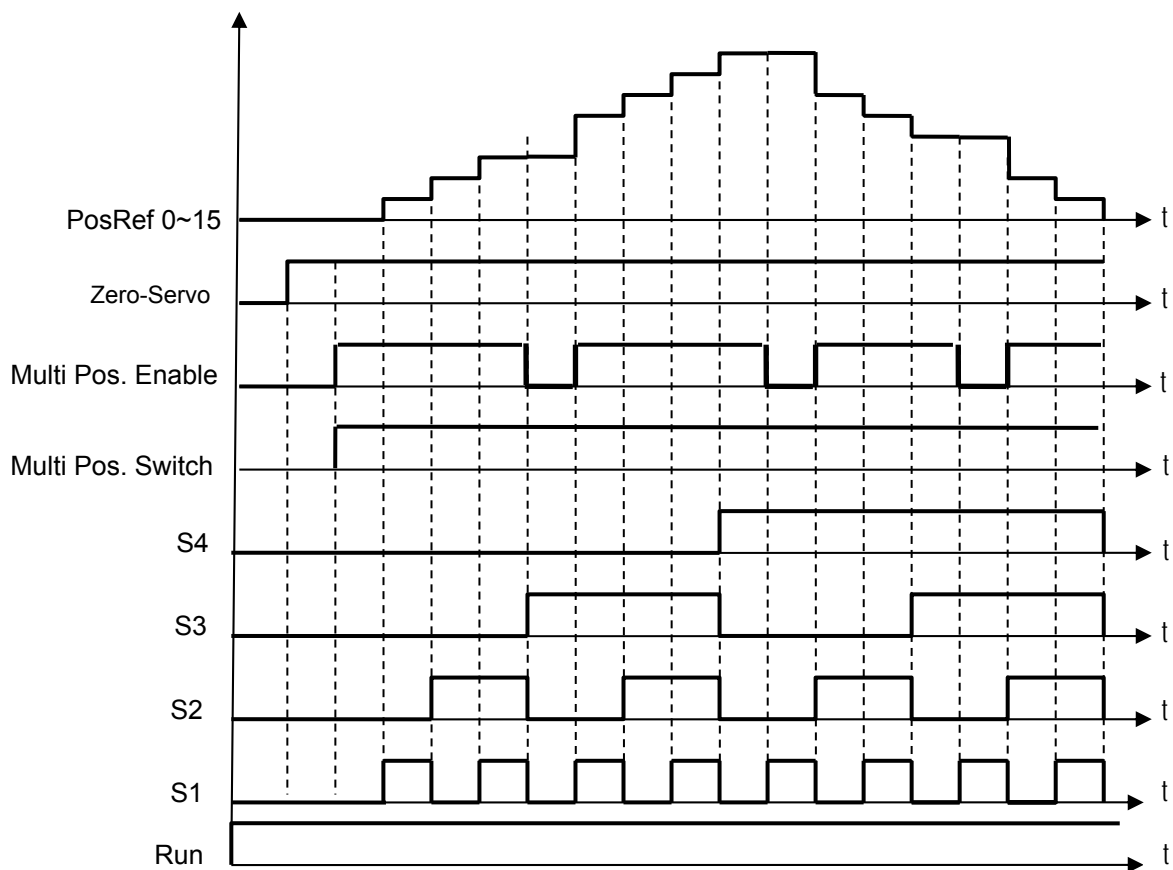
圖 4.3.130 多點定位功能示意圖
