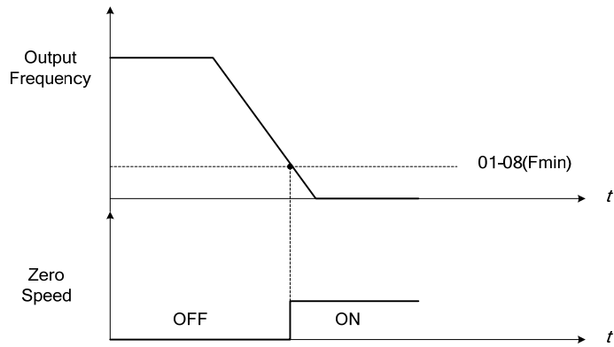
圖4.3.26 零速度操作
