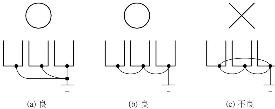
圖 3.6 A510s 多台接地方法
