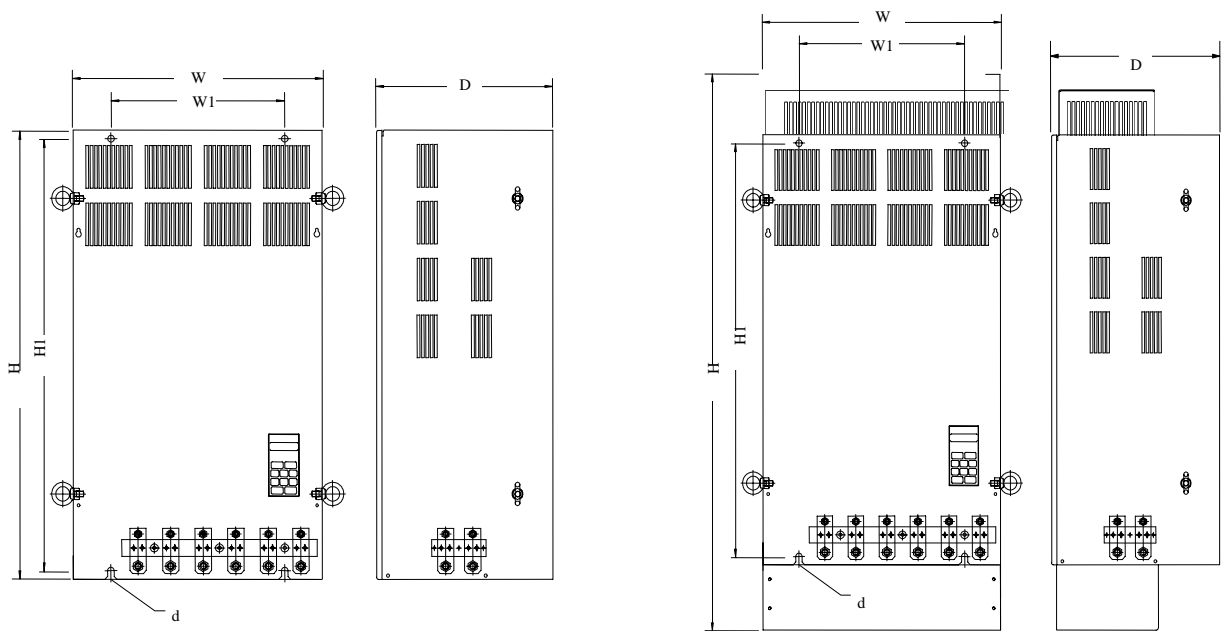
( 盤內安裝型 - IP00 )
