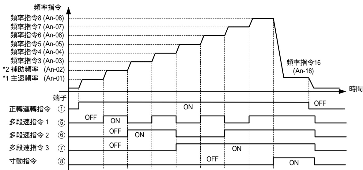
圖 42 16 段速運轉控制
