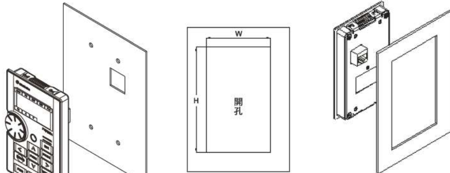
盤面安裝開孔尺寸圖：
